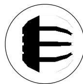
DynamoDB
