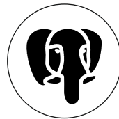
PostgreSQL
